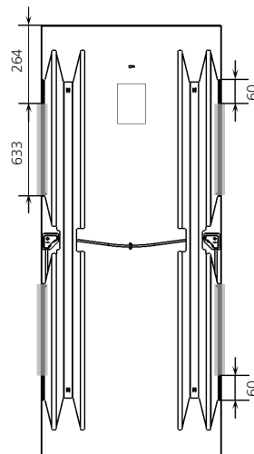
Abb. 2 Rückseite Modul
